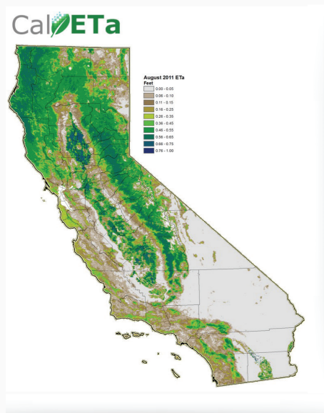
— FIGURE A10. ETa Map Year 2011
